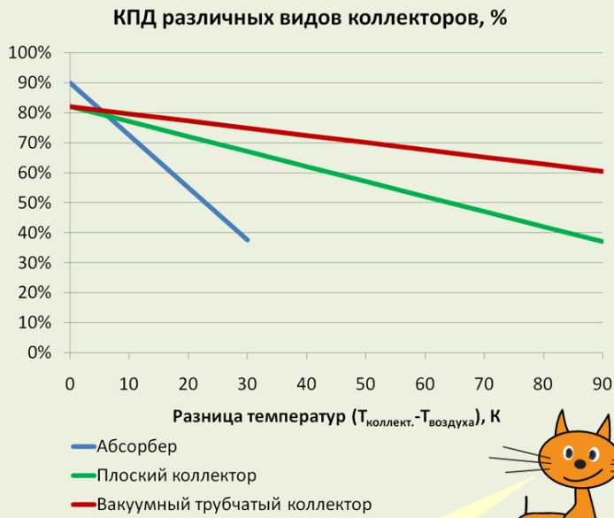
Вакуумный трубчатый коллектор
