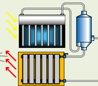
Вакуумный трубчатый коллектор
