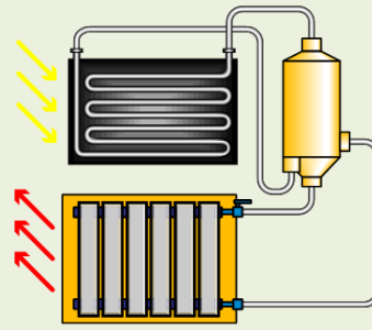
Плоский коллектор
